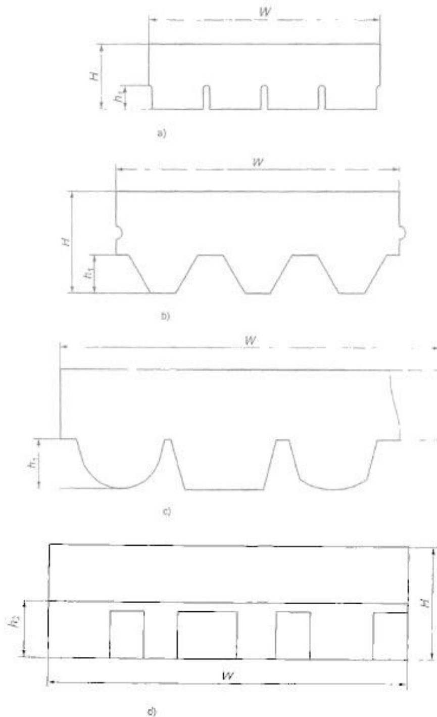
а, б, в) – Примеры однослойной черепицы; д) – Пример многослойной черепицы
