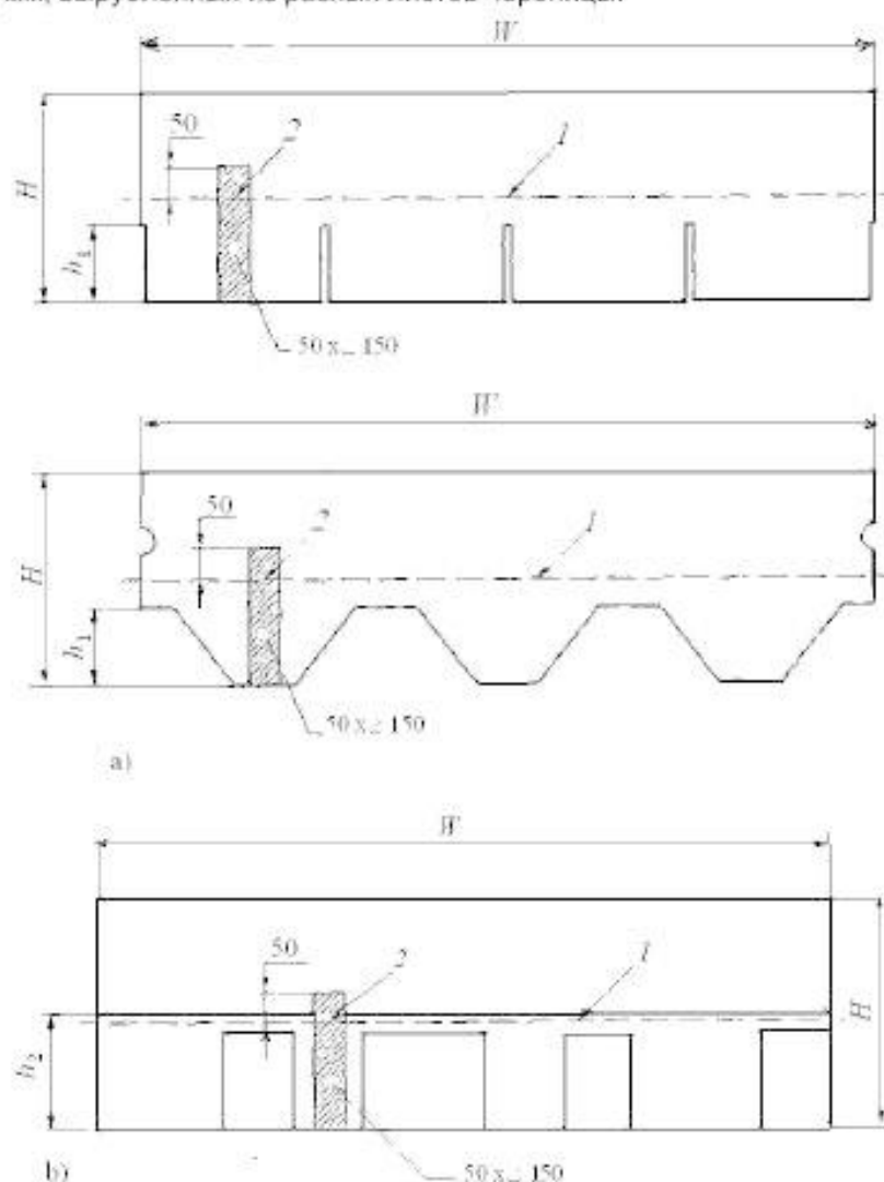
а) – Положение гвоздя для однослойной черепицы; б) – Положение гвоздя для многослойной черепицы H – высота листа; W – ширина листа; h_1 – высота прорезей; h_2 – высота нижнего слоя 1 – положение гвоздя в соответствии с инструкцией по укладке (см. 5.5); 2 – положение гвоздя в образце
