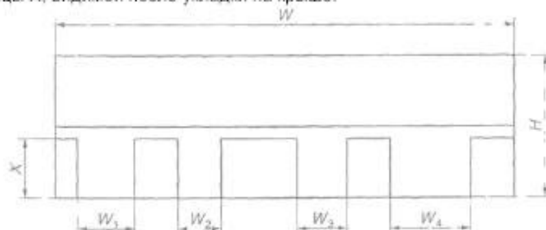
Рисунок 6 – Определение площади нахлеста для многослойной черепицы
