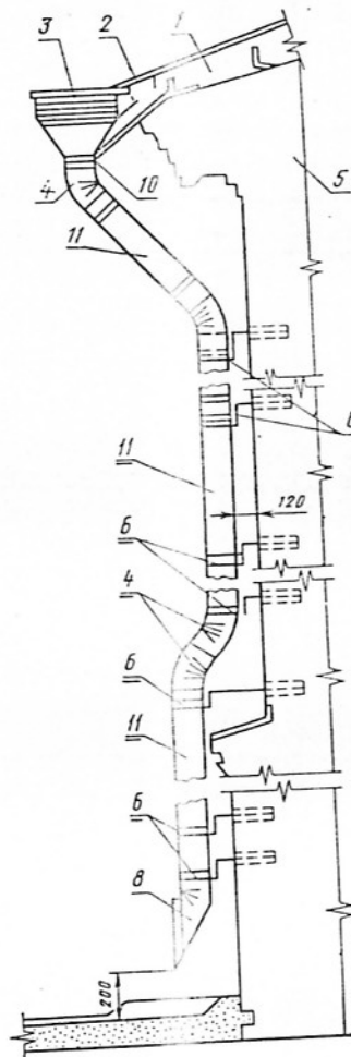
Применение звеньев труб типов ТВ1 и ТВ2
