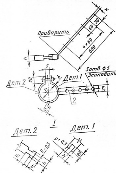
Хомут с планкой типа ХП
