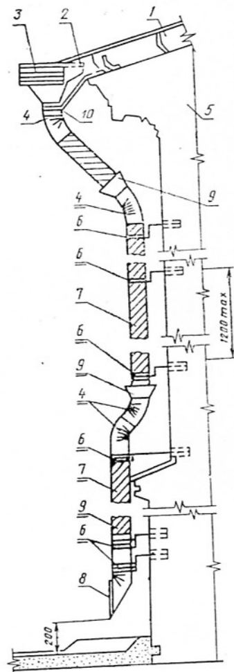
Применение звеньев труб типа ТС
