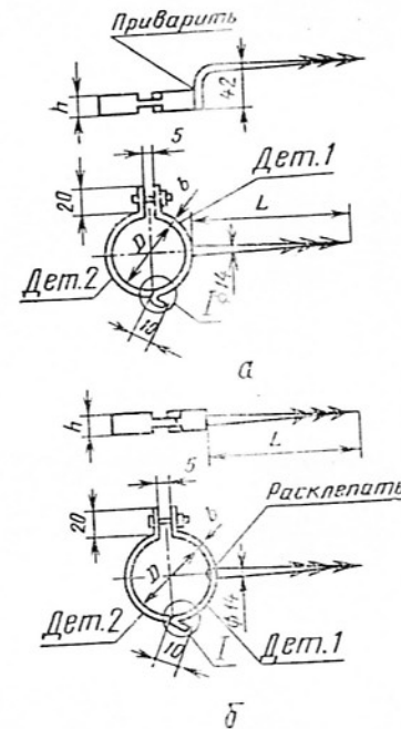
Хомут со штырем типа ХШ
