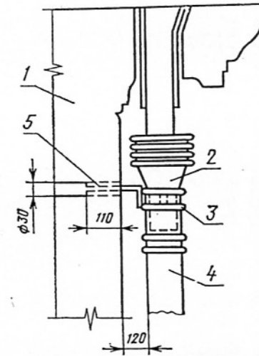
Крепление подкарнизной воронки
